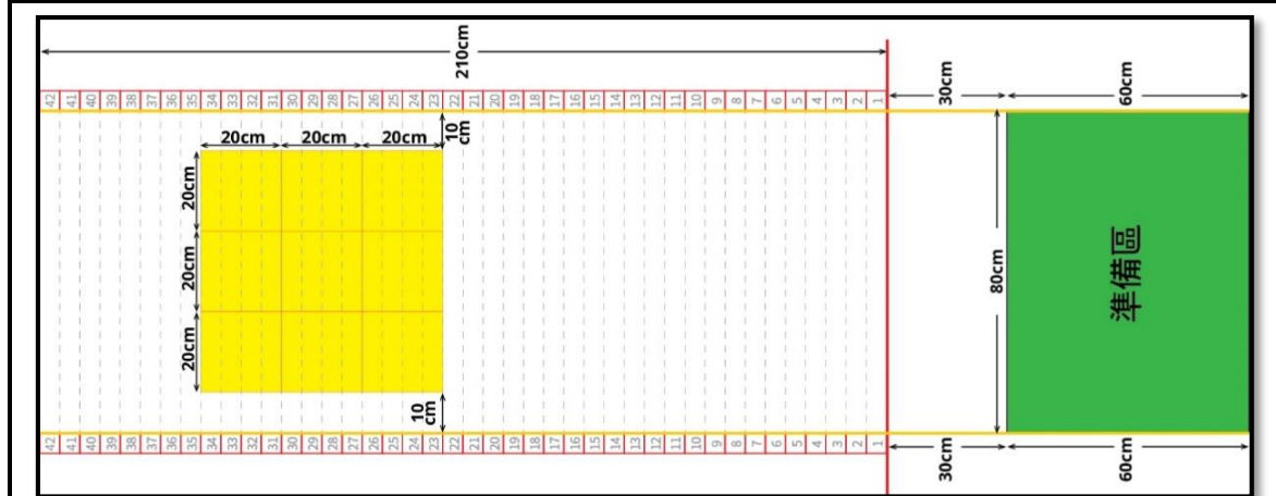
圖 9-3 競賽用場地尺寸標示
